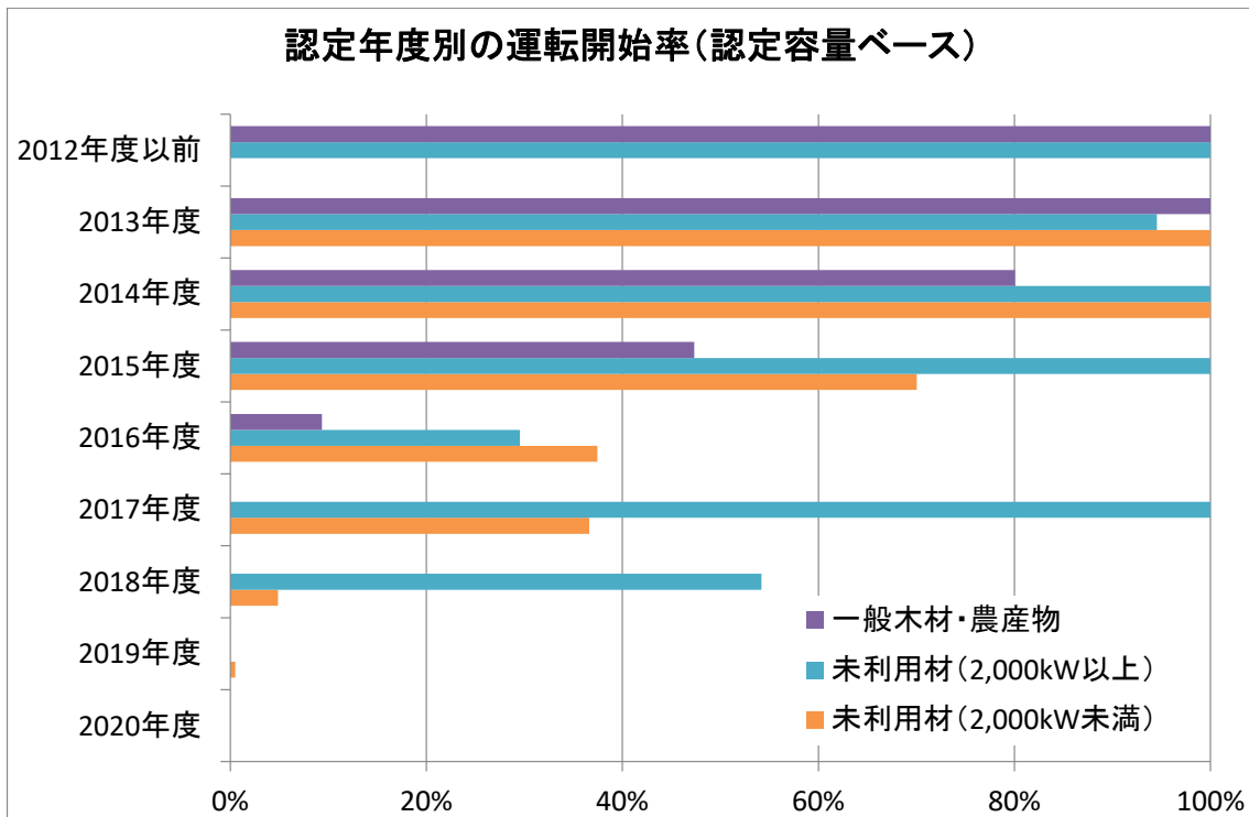
(出典) 経済産業省公表資料(2020年6月時点)に基づいて独自集計 図3 木質バイオマス・農産物残さの認定年度別運転開始率(認定容量ベース)
