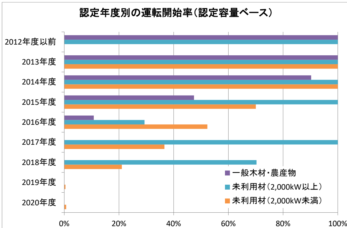
(出典) 経済産業省公表資料(2020年12月時点)に基づいて独自集計 図3 木質バイオマス・農産物残さの認定年度別運転開始率(認定容量ベース)
